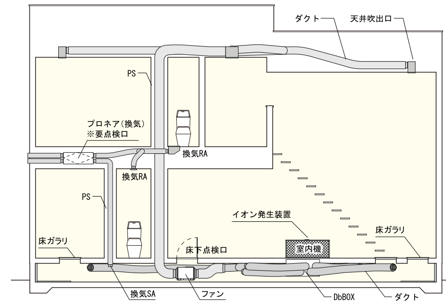
概念断面図
